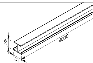
Tragprofil H31 S19-TP-004
