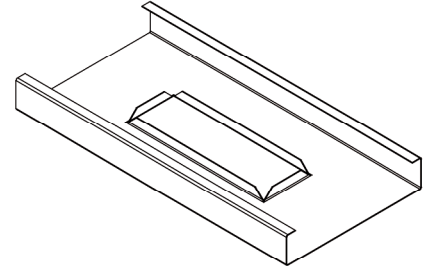
Ausschnitt Typ 2 Q mit Aufkantung, mit Verstärkungswinkel quer
