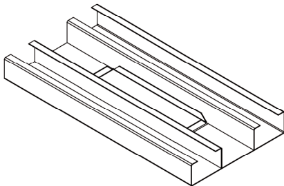
Ausschnitt Typ 2 L mit Aufkantung, mit Verstärkungswinkel längs
