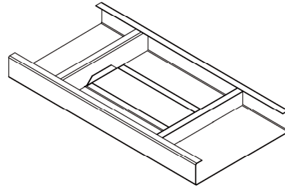
Ausschnitt Typ 2 Q mit Aufkantung, mit Verstärkungswinkel quer
