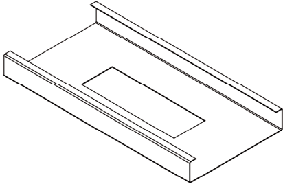
Ausschnitt Typ 2 L mit Aufkantung, mit Verstärkungswinkel längs
