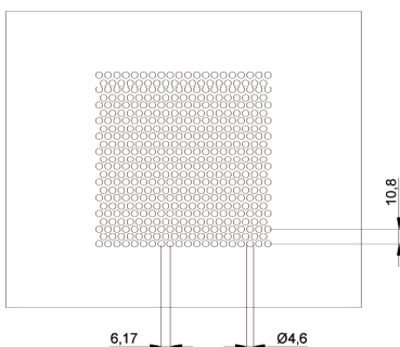
Lautsprecher- oder Lüftungsperforation Typ 3
