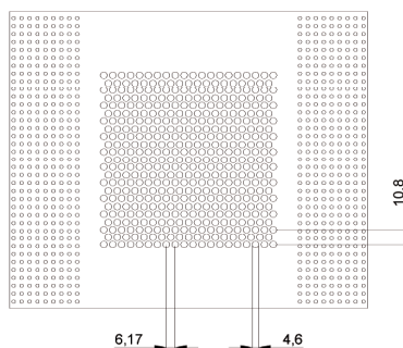
Lautsprecher- oder Lüftungsperforation Typ 5
